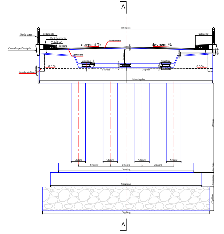
COUPE B-B DE LA CULEE C0 ECH
